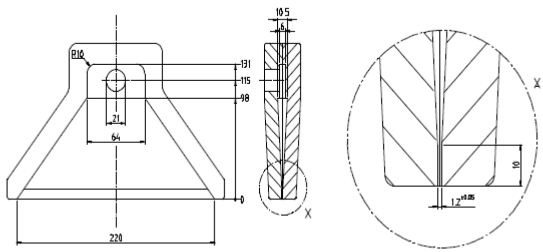
图 31：浪涌水试验—浪涌喷嘴
