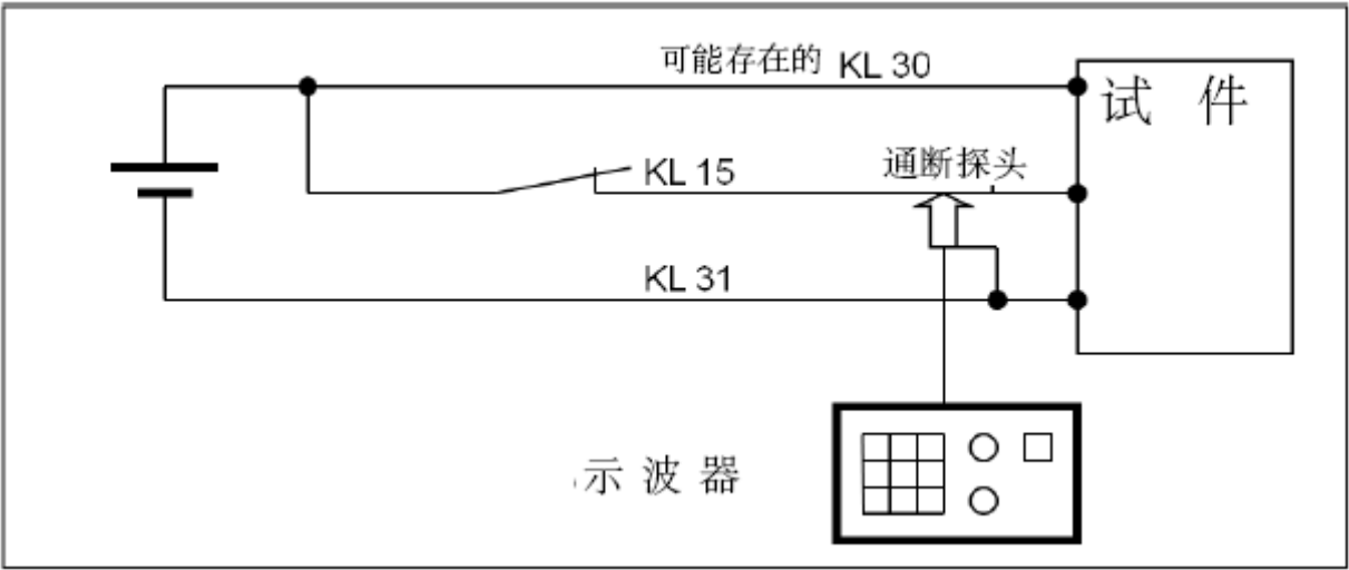
图 17: E-21 反馈试验接线原理图
