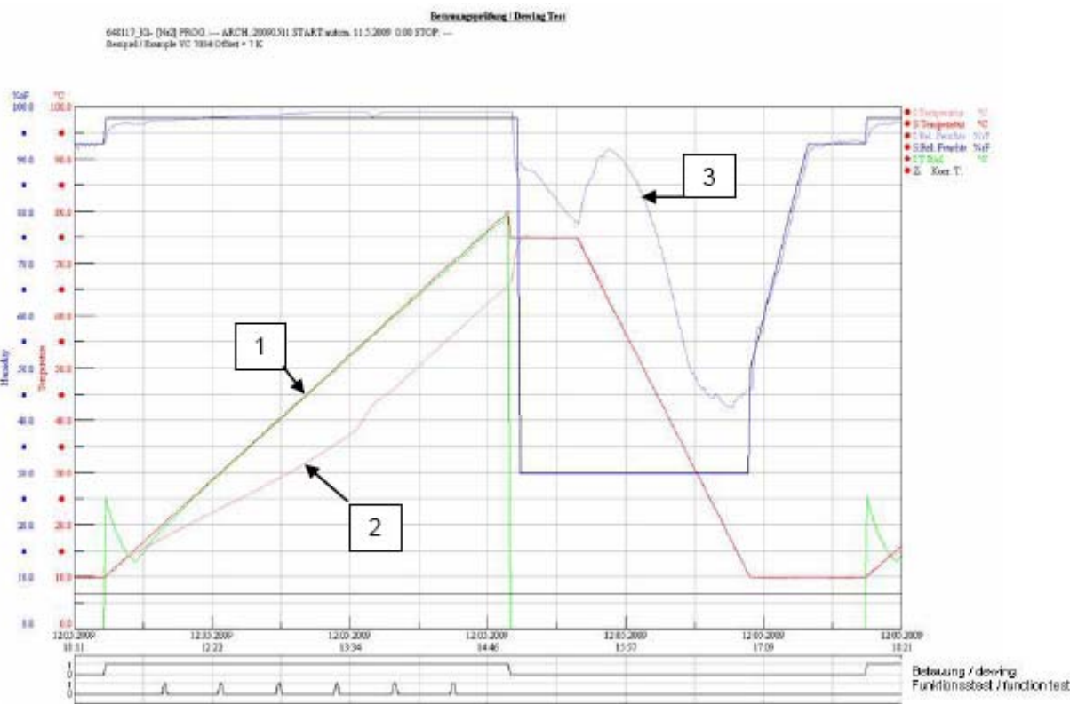
图 44：凝露试验流程，一次循环
