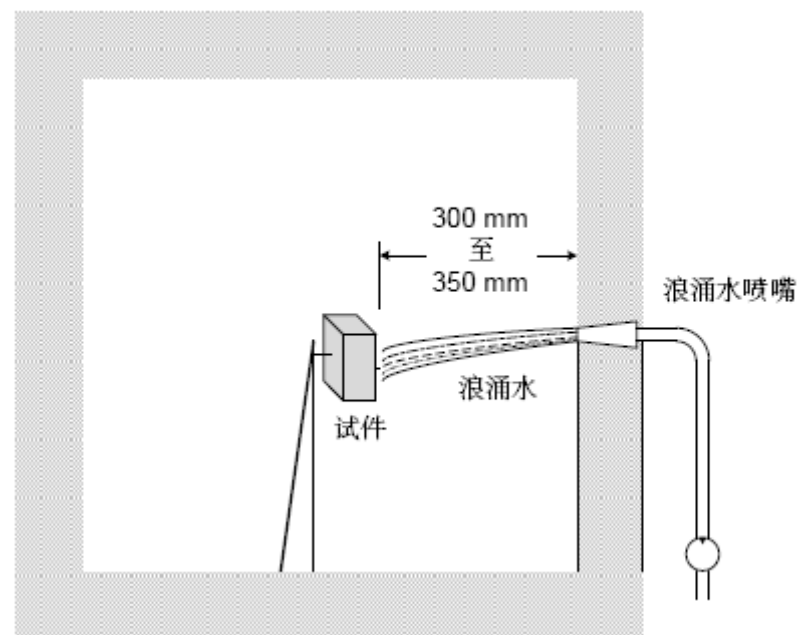
图 32：浪涌水试验结构
