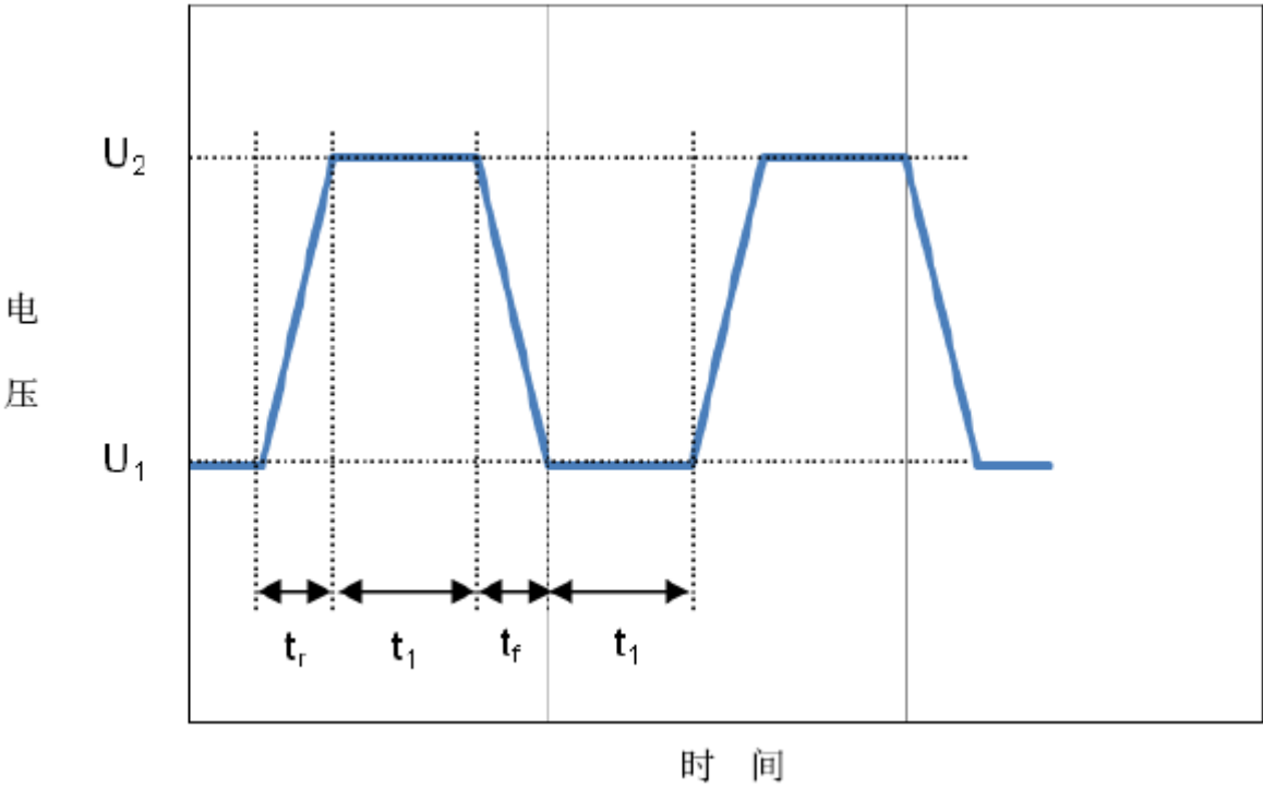
图 13: E—12 具有智能发电机调节装置的电压波动波形试验脉冲
