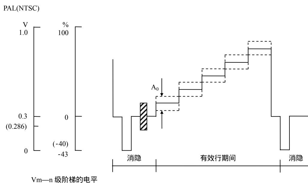
图 24 微分增益测试信号图
