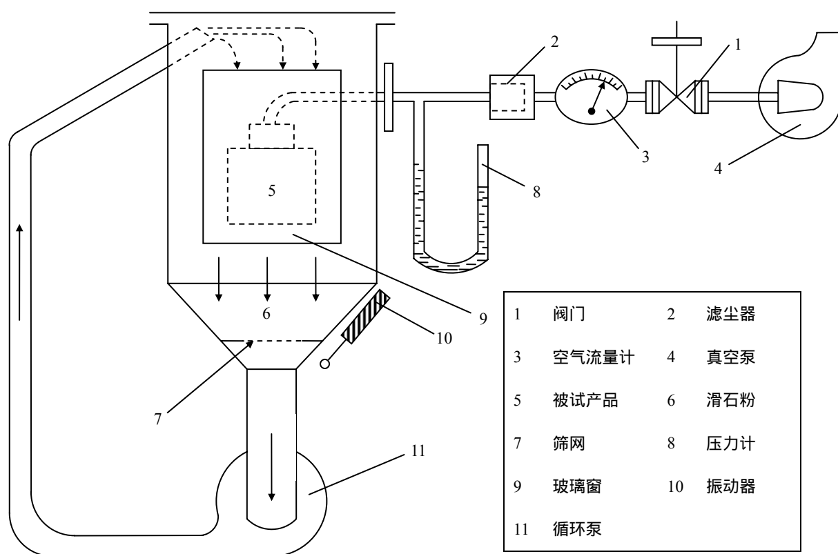
图A - 2 粉尘试验用的试验柜的结构示
