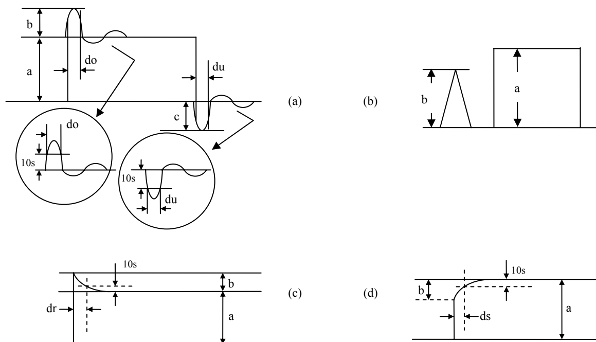
图 14 亮度波形失真图
