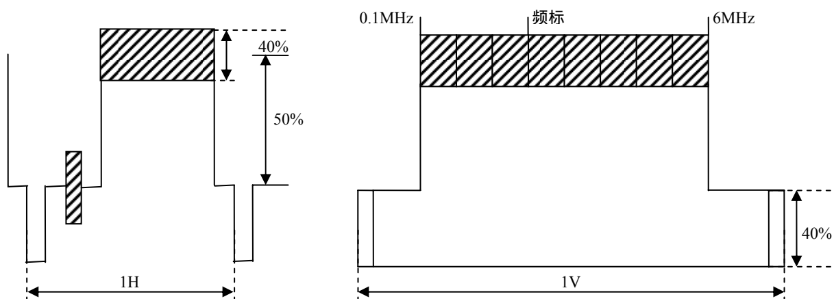
图 11 复合视频测试信号
