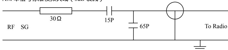
b) AM 双信号标准模拟天线 (-6dB 衰减)
