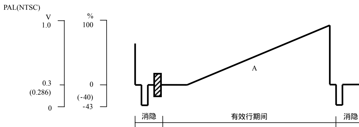
图 16 亮度信噪比测试信号
