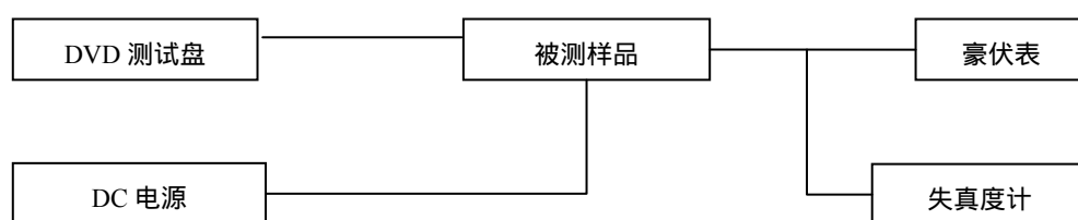
图 36 测试原理图
