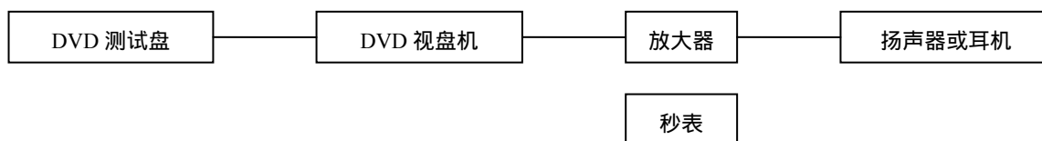
图 35 读取时间测试方框图
