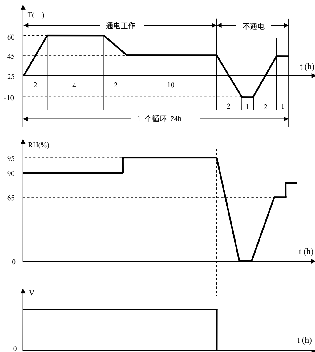
图1 温度、湿度交变曲线
