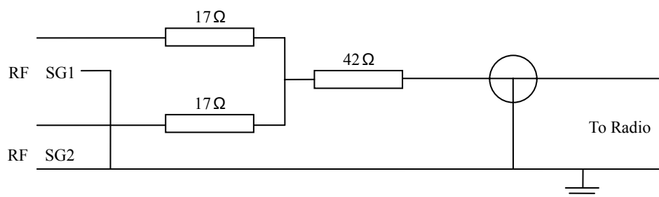
图5 FM 标准模拟天线
