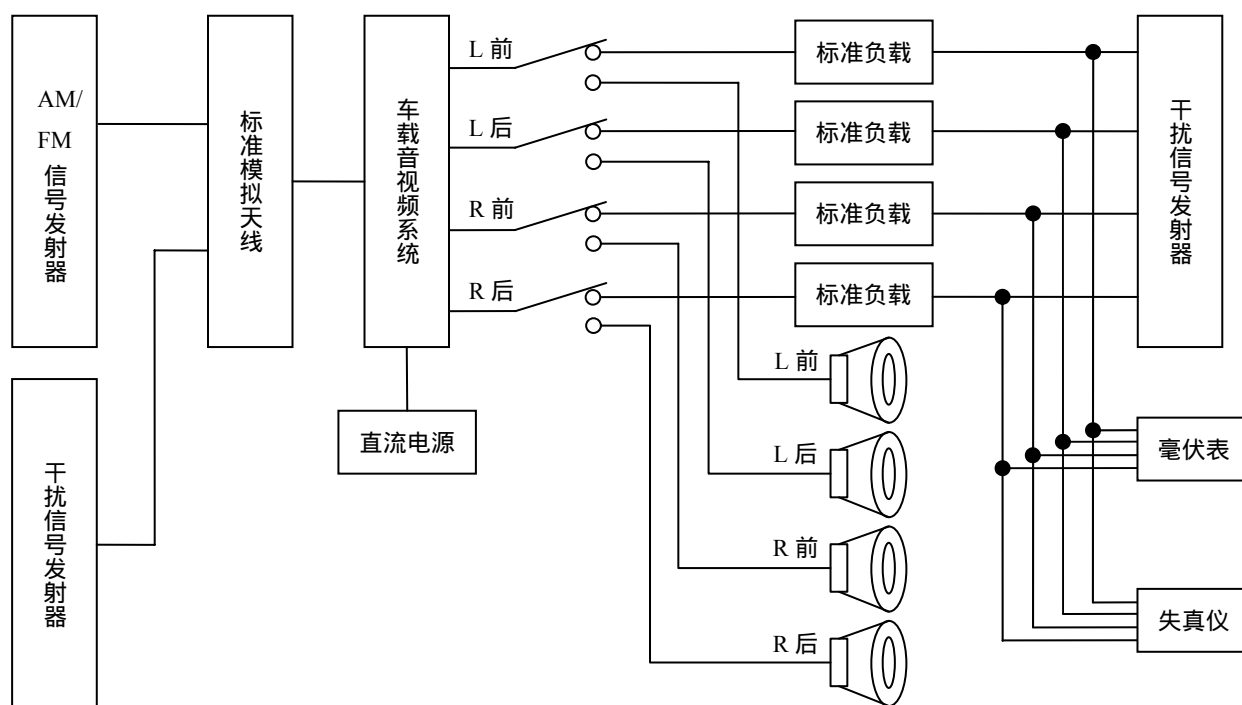
图 4 AM/FM 接收机电性能测试连接示意图
