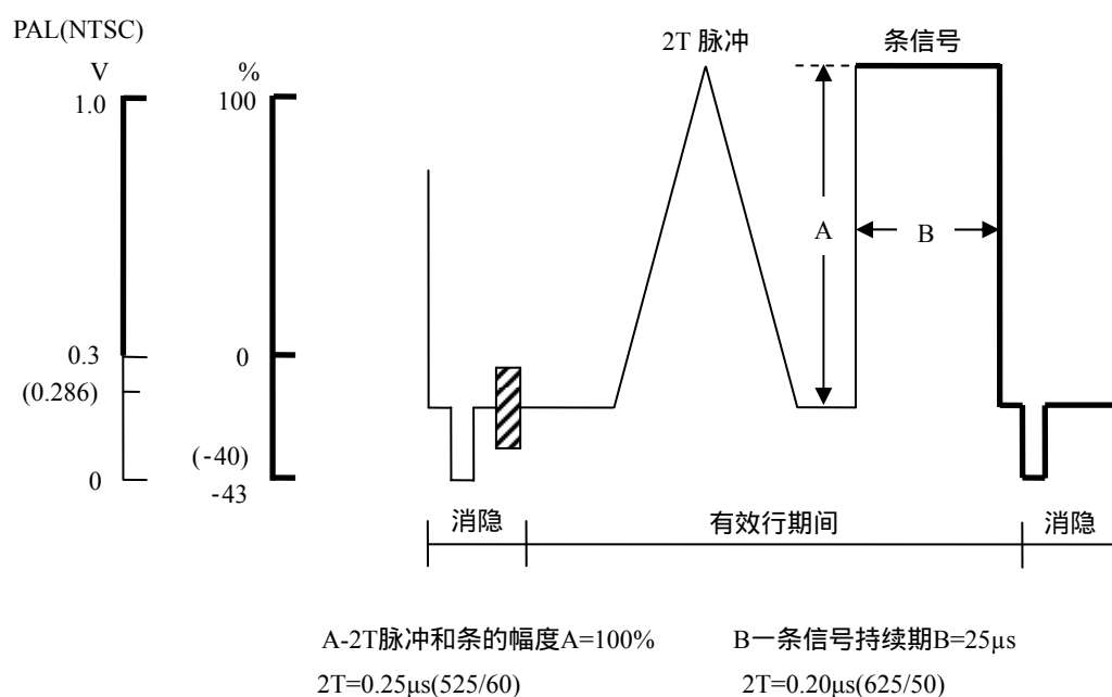
图 13 亮度波形失真(线性)测试信号图
