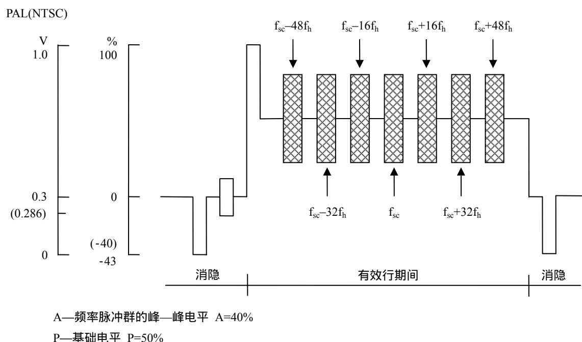
图 17 色度幅频响应测试信号
