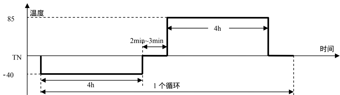
图2 热冲击试验曲线
