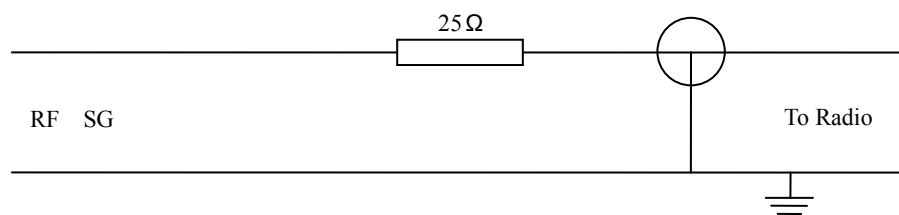
b) FM 双信号标准模拟天线 (-6dB 衰减)
