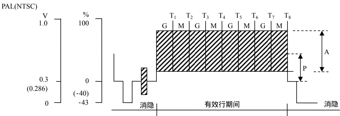
(a) 全场信号
