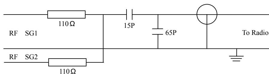
b) AM 双信号标准模拟天线 (-6dB 衰减)
