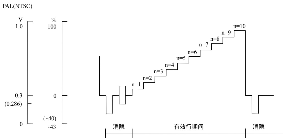
图 12 亮度非线性失真测试信号(10 级)
