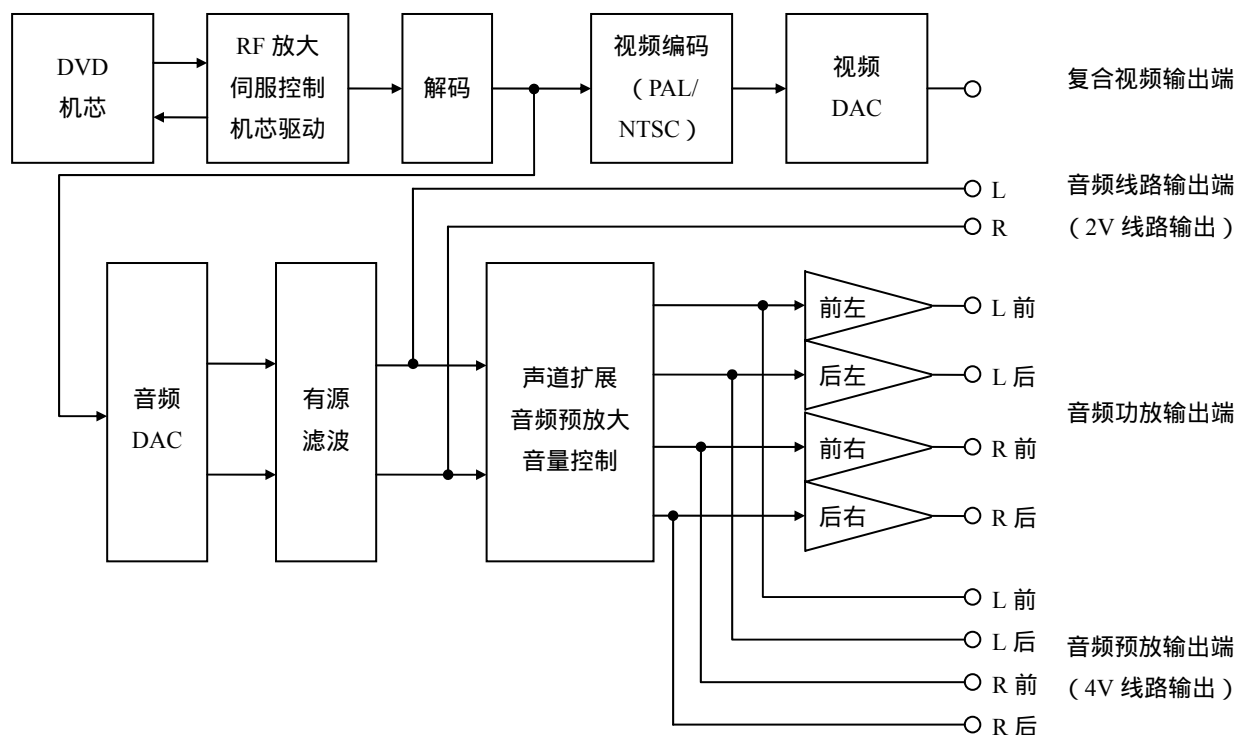
图 A - 1 DVD 音视频输出端在整机线路中的参考位置
