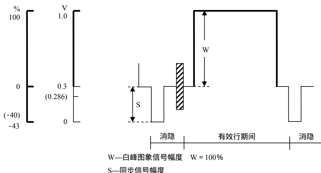
图9 视频测试信号图
