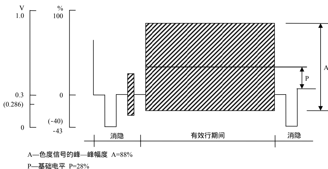
图 19 色度信噪比测试信号
